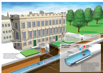
1 - Récupérateur de calories servant à chauffer et rafraîchir le Muséum rénové
